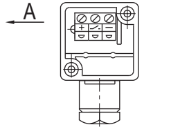
Маркировка клемм
