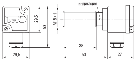
Габаритный чертеж
